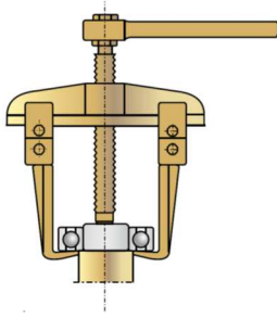
Рисунок 7.4. Съемник подшипников качения
