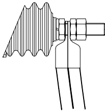
Рисунок 4.6. Подключение параллельных кабелей
