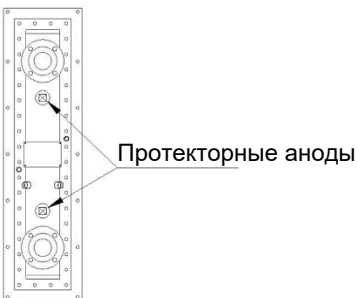
Рисунок 4.4. Радиатор с протекторными анодами
