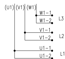
Рисунок 4.7. Параллельные соединения
