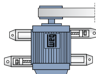
Рисунок 4.10. Скользящее основание
