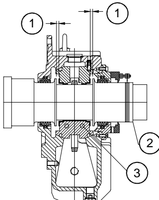
Рисунок 4.17. Подшипник скольжения
